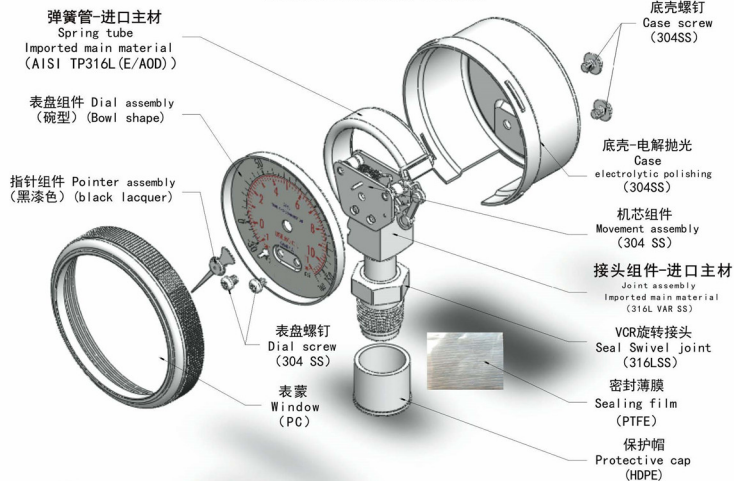
产品分解示意图 Product Breakdown Diagram
